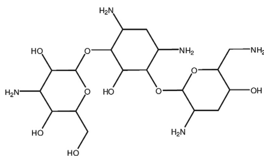
Tobramycin
