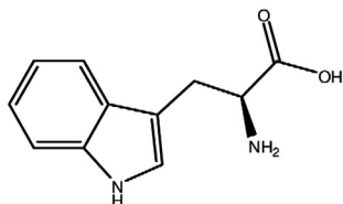
L-tryptophane
