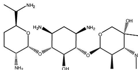
Gentamicin
