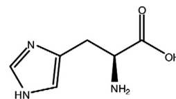
L-histidine
